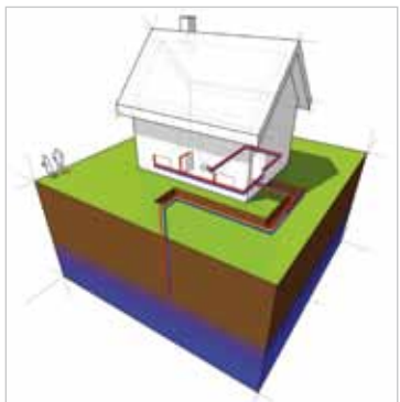
Geotermia. | QUENERGIA.COM
