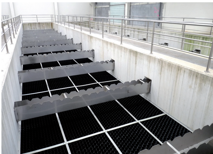
Lokatza tratatzeko instalazioak.
