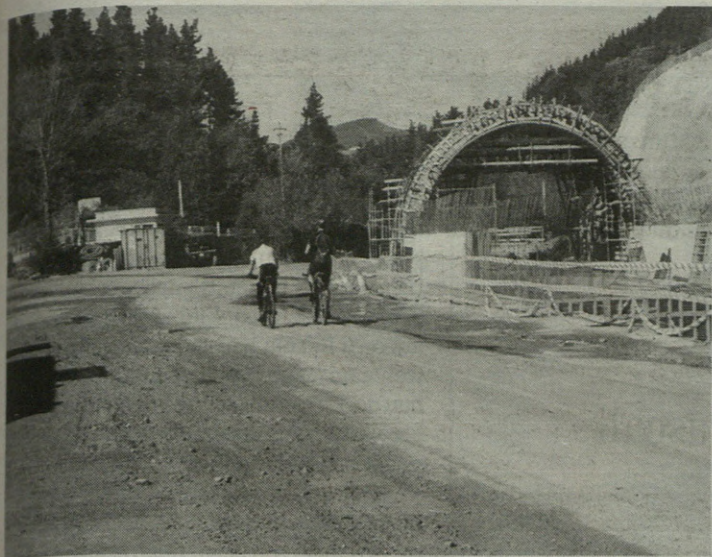
ANGIOZARKO TUNELA. Bergaratik Angiozarrera bidean eraikitzen ari diren tunela zeharkatu beharko dugu. Autobidea gainetik doa.
