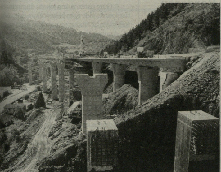
IPINARRIKO ZUBIBIDEA. Bergarako irteeran Arrasate eta Eibar arteko zubibiderik luzeena eraikitzen ari dira, 640 metrokoa.
