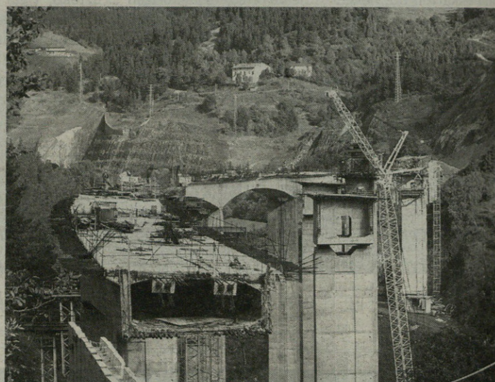
LARREATEGIKO ZUBIBIDEA. Soraluze eta Maltzaga artean dago eta Deba ibarra aldenik alden zeharkatuko du. 400 metro luze.
