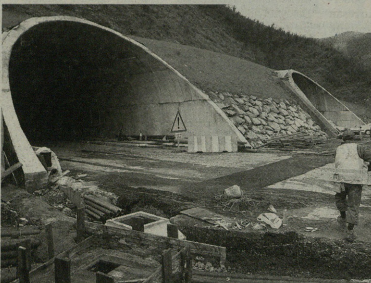
GALLASTEGIKO TUNELA. Eibar-Arrasate zatiko tunelik luzeena (2,4 kilometro). Autobideko luzeena, berriz, Arlabangoa izango da.
